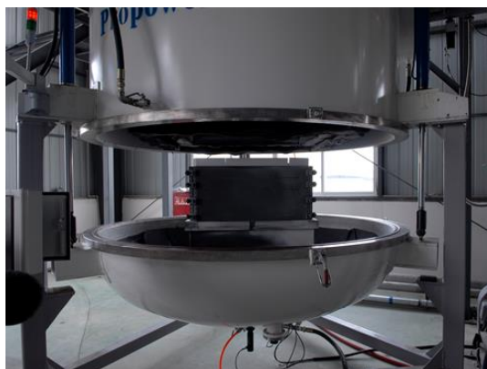
多晶硅铸锭生产设备
