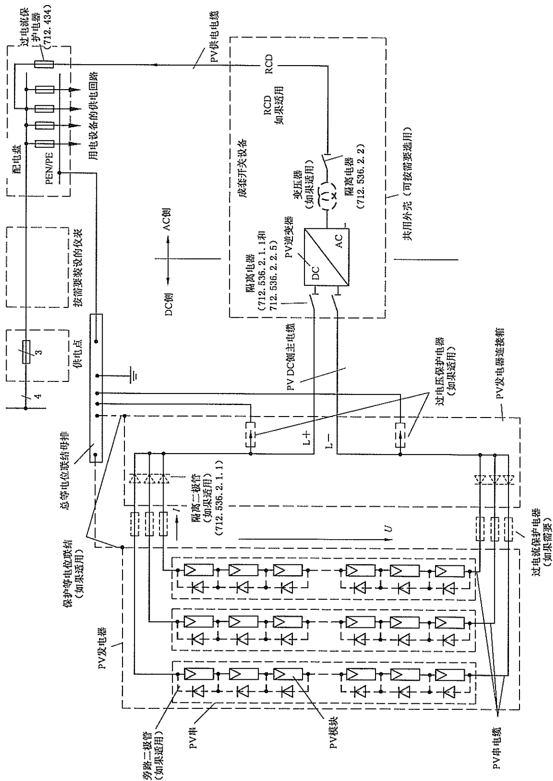
图 712.1 PV 装置——概略总图(单个阵列)
