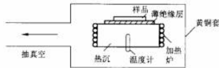
图1 样品架示意图
